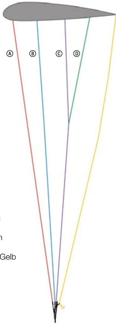
3.1. Flügelprofil des KUDOS 2
